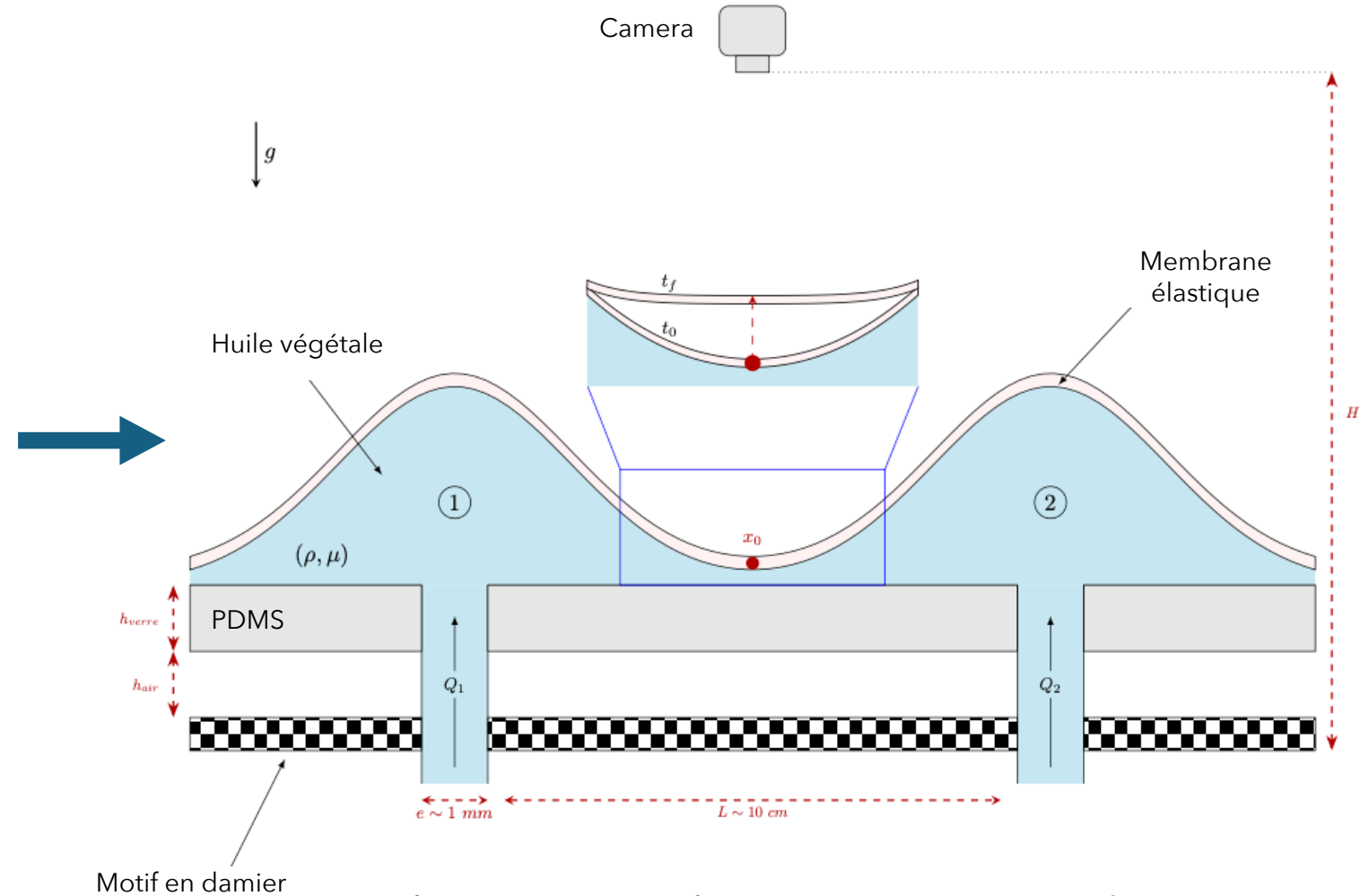
Schématisation du setup expérimental
