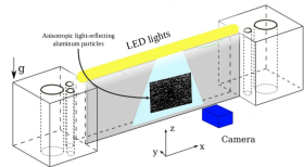
Visualisation setup
