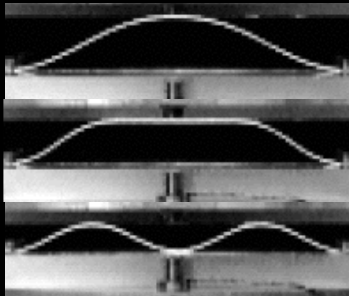
[Roman & Pocheau 99]
