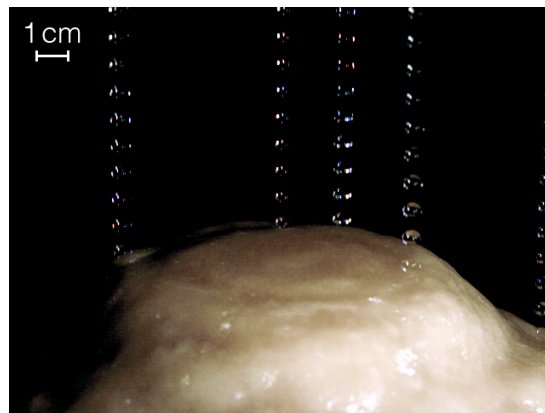
Figure 1. Les gouttes tombant d'une stalactite n'atterrissent pas au même endroit sur la stalagmite située dessous. Montage de vidéos prises à Orgnac (France), images séparées de 740 \mu s. Crédit : The Royal Society 2019 [2].
