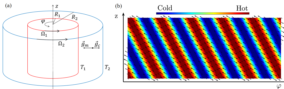
Figure 1. Représentation schématique du système (a) et profils de vitesse et de température dans le plan azimuthal/axial ( \varphi, z ) d'une instabilité thermomagnétique sans rotation des cylindres (b).
