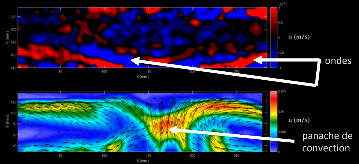
Visualisation de l'écoulement par PIV coupe verticale
