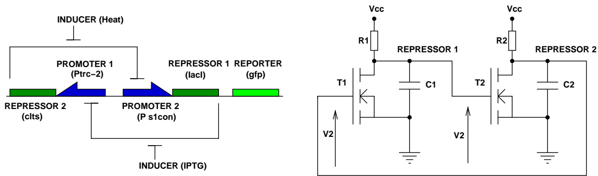
Fig.4. Dans la figure a, nous représentons le schéma logique du toggle-switch publié par Gardner et al. . La figure b représente le schéma électronique du toggle-switch conçu avec deux transistors.
